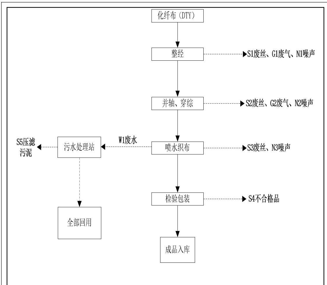
图2-3 雨伞布生产工艺流程及产污节点图
