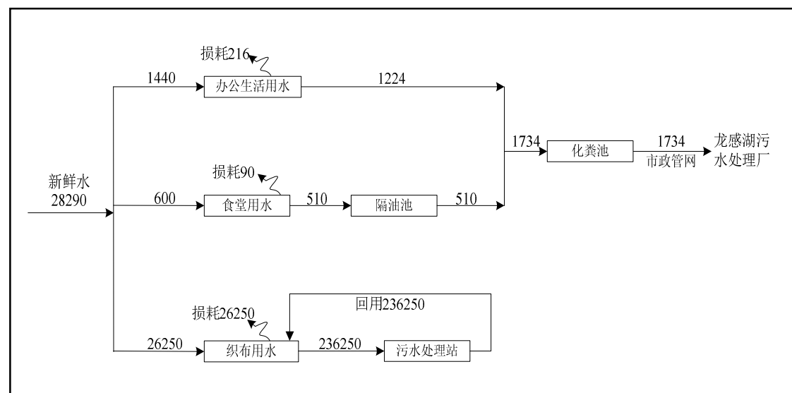
图2-1 水平衡图（m 3 /a）
