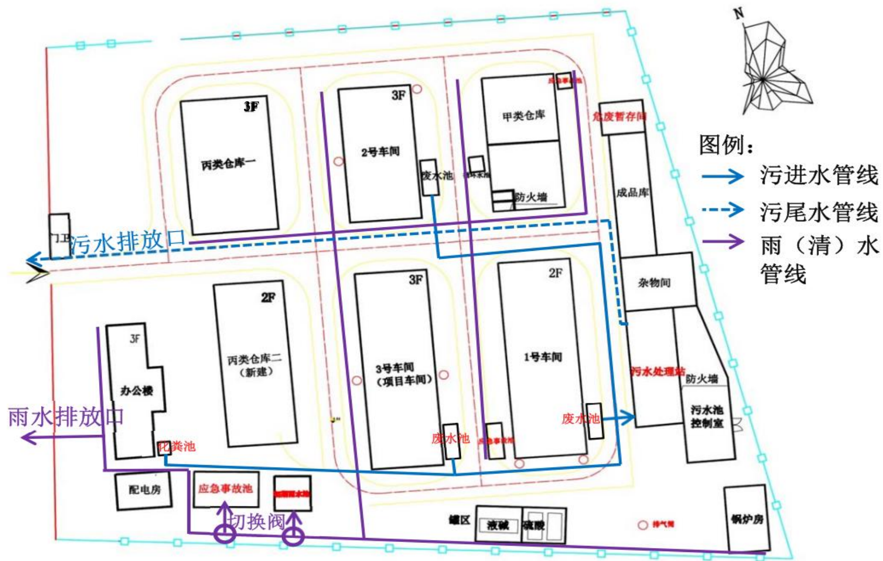
附图 4 项目雨污管网图
