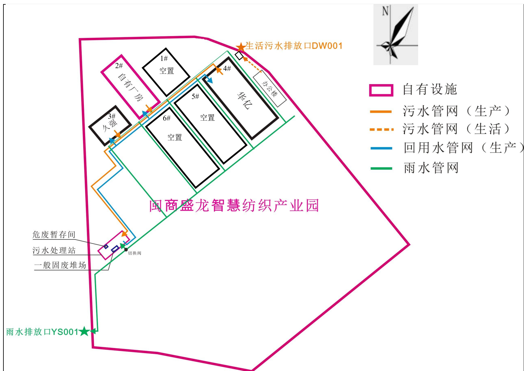
附图3 项目平面布置图及雨污管网图
