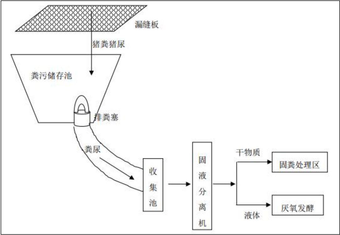
图 3.5-3 项目污粪处理工艺流程图
