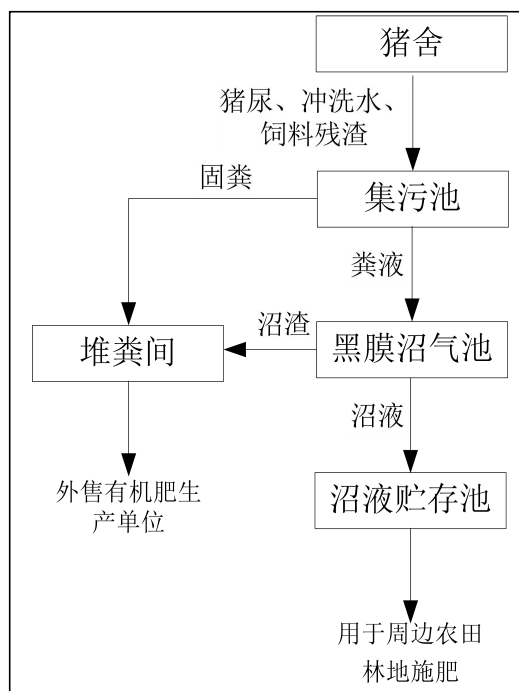
图 4.1-1 废水处理工艺流程图
