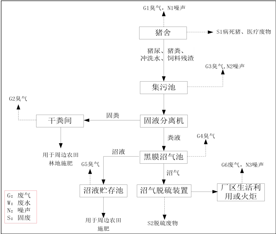
图 3.5-2 饲养工艺流程及产污节点图
