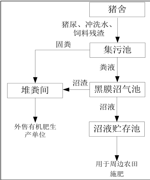
图 3.5-4 项目污水处理工艺流程图
