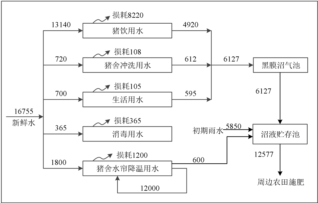
图 3.4-1 项目水平衡图（单位：m³/a）
