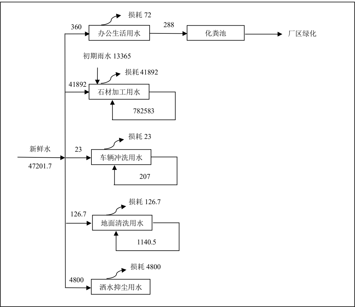
图 2-2 项目水平衡图 (单位: m³/a)
