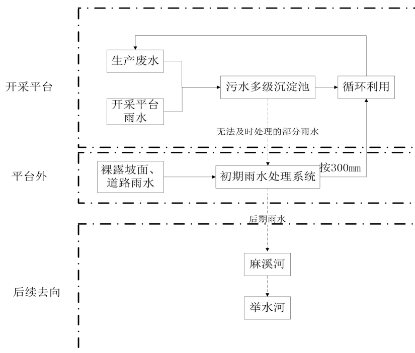
图 4-5 本项目排水流程示意图
