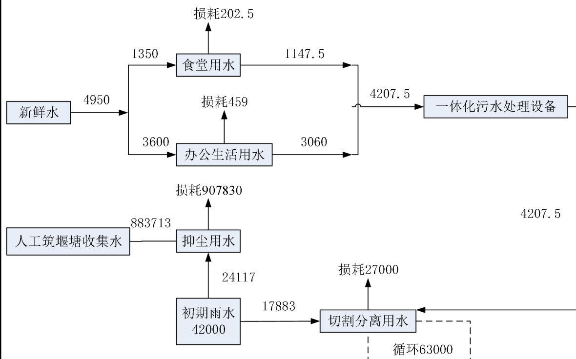
图 4-3 项目年水平衡图 单位: m 3 /a
