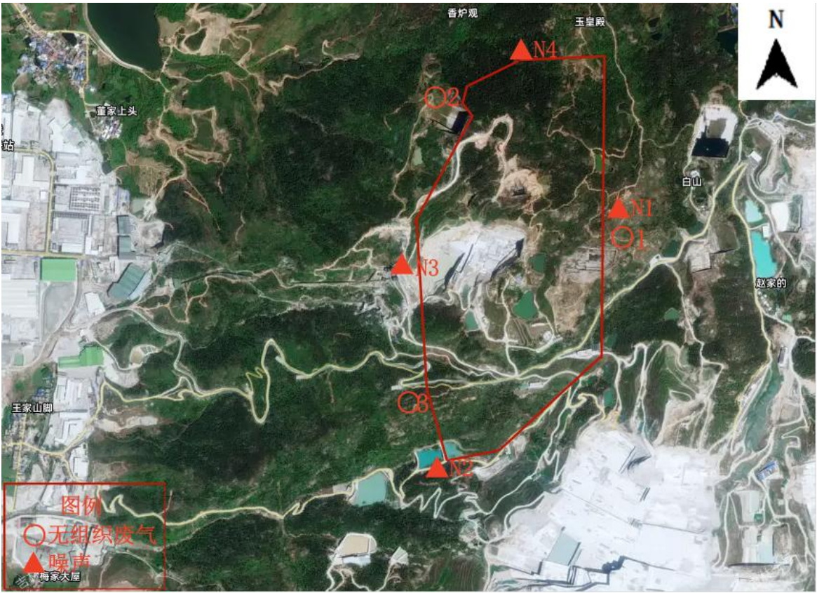
图 8-1 项目监测点位布置图
