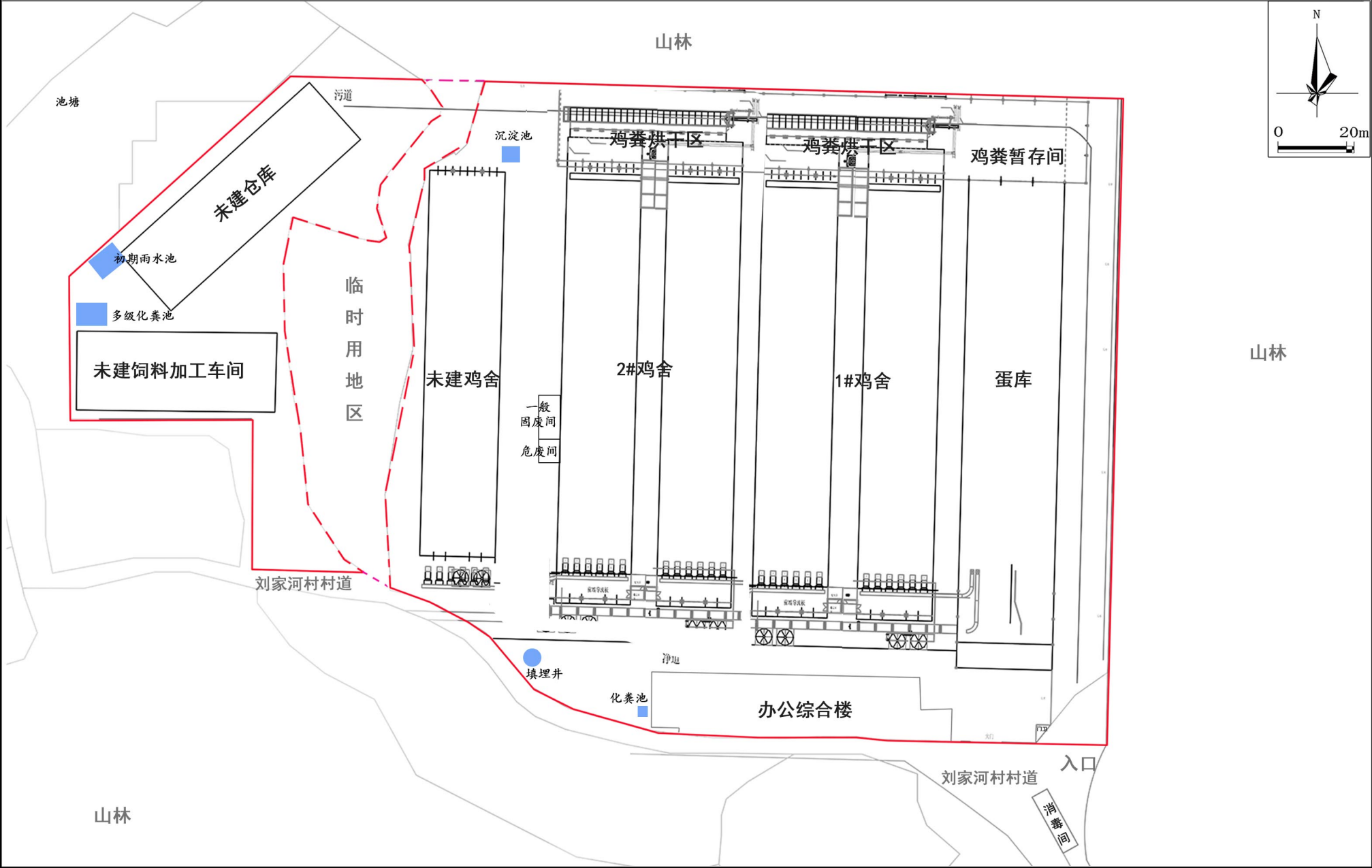
附图3 验收阶段总平面布置图
