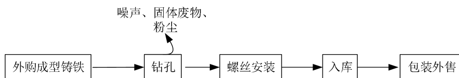
图 2-3 项目烧嘴生产工艺流程及产污节点图
