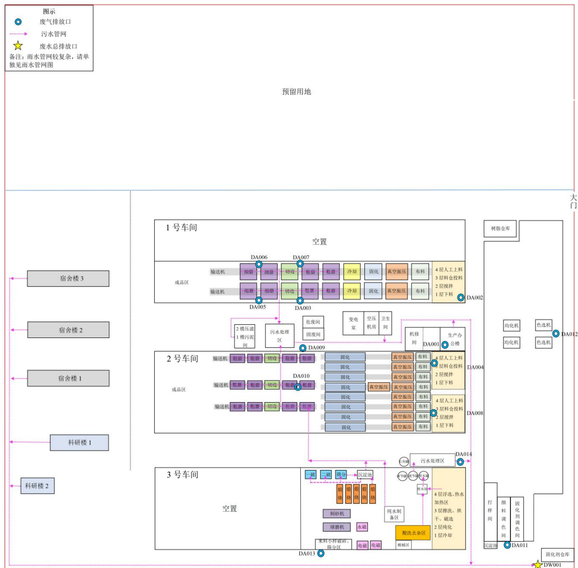
附图 4 平面布置图 (含污水管网)
