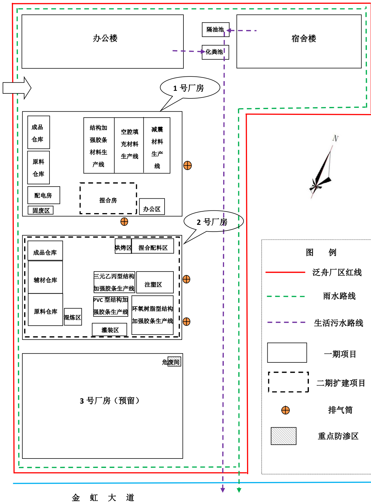
附图3 本次扩建项目厂区平面布置图
