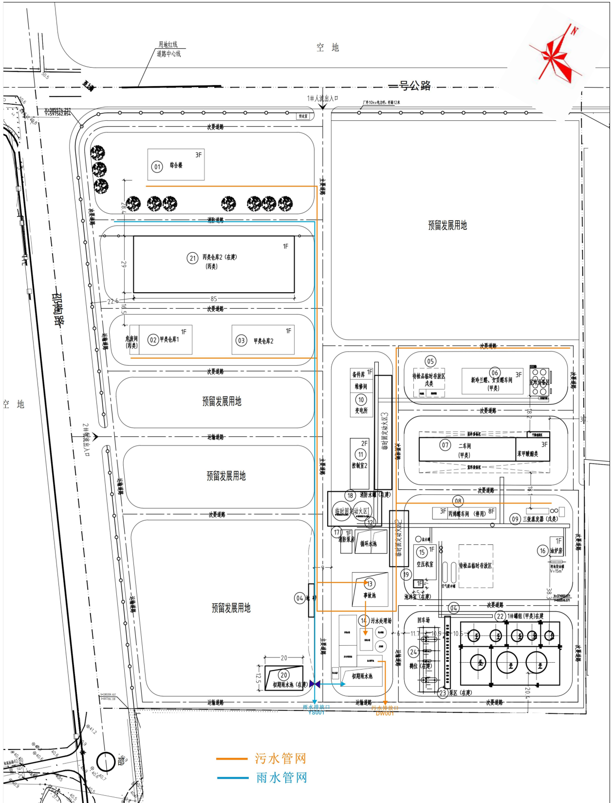
附图4 项目厂区雨污管网图
