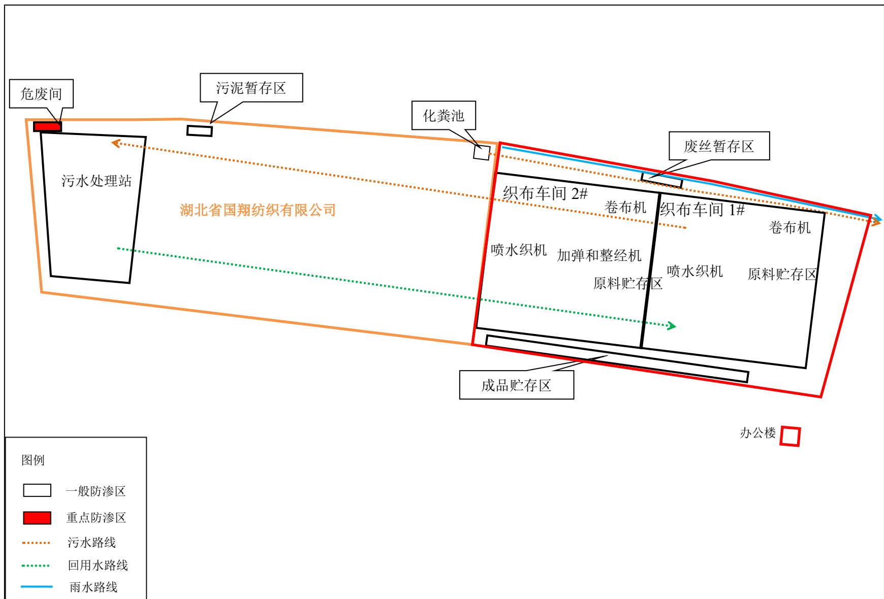
附图 3 项目平面布置图及雨污管网图
