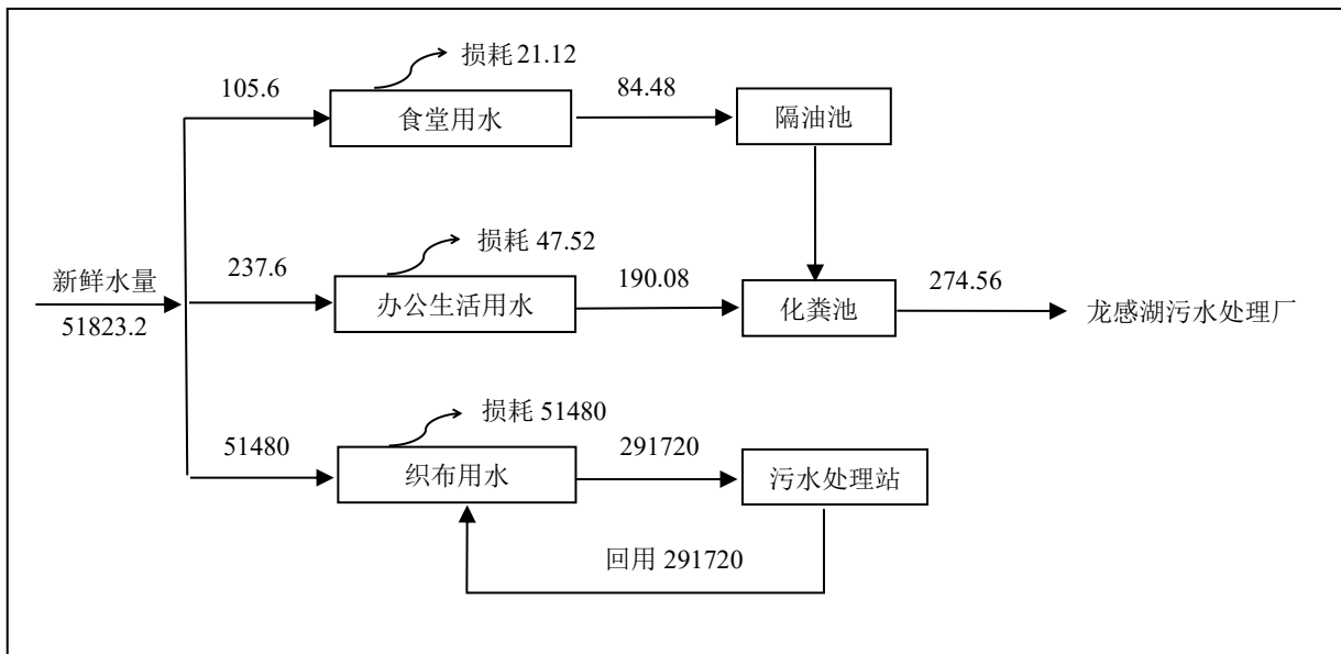
图 2-2 项目水平衡图 (单位: \text{m}^3/\text{a} )
