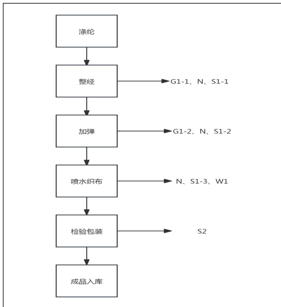
图 2-3 生产工艺流程及产污节点图
