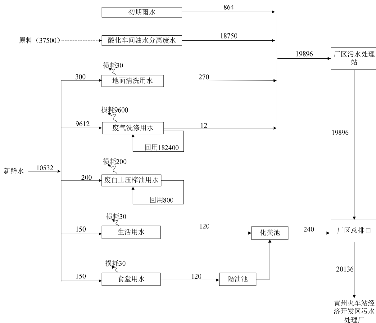
图 3-5 项目水平衡图 (单位: m³/a)
