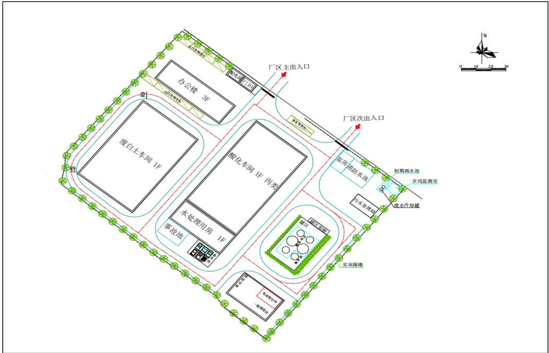
图3-4 项目总平面布置图
