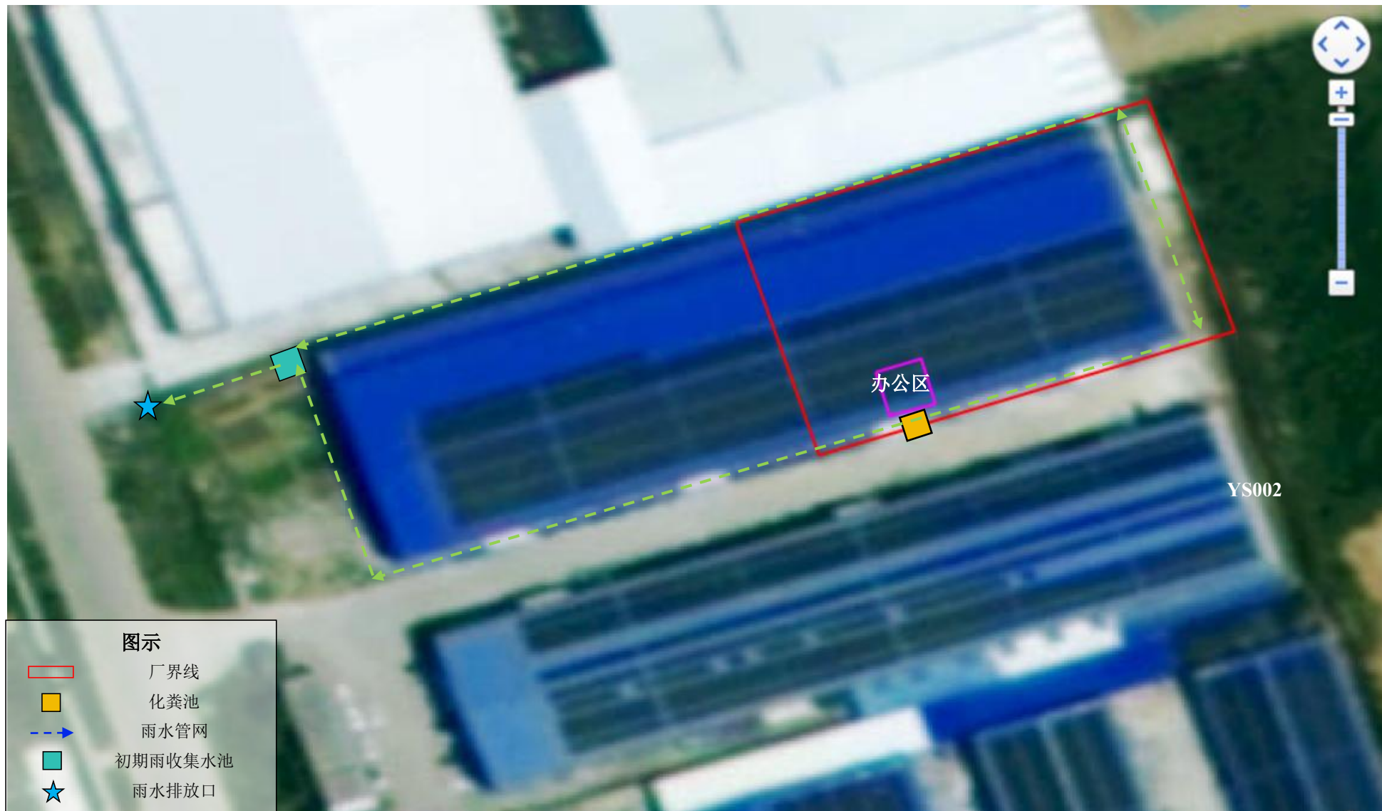
附图 4 项目雨水管网图
