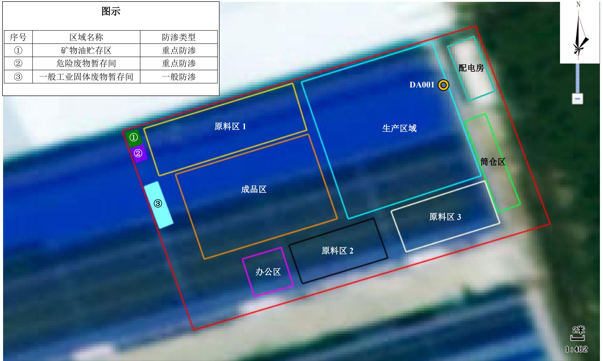
附图 3 项目平面布置及分区防渗图
