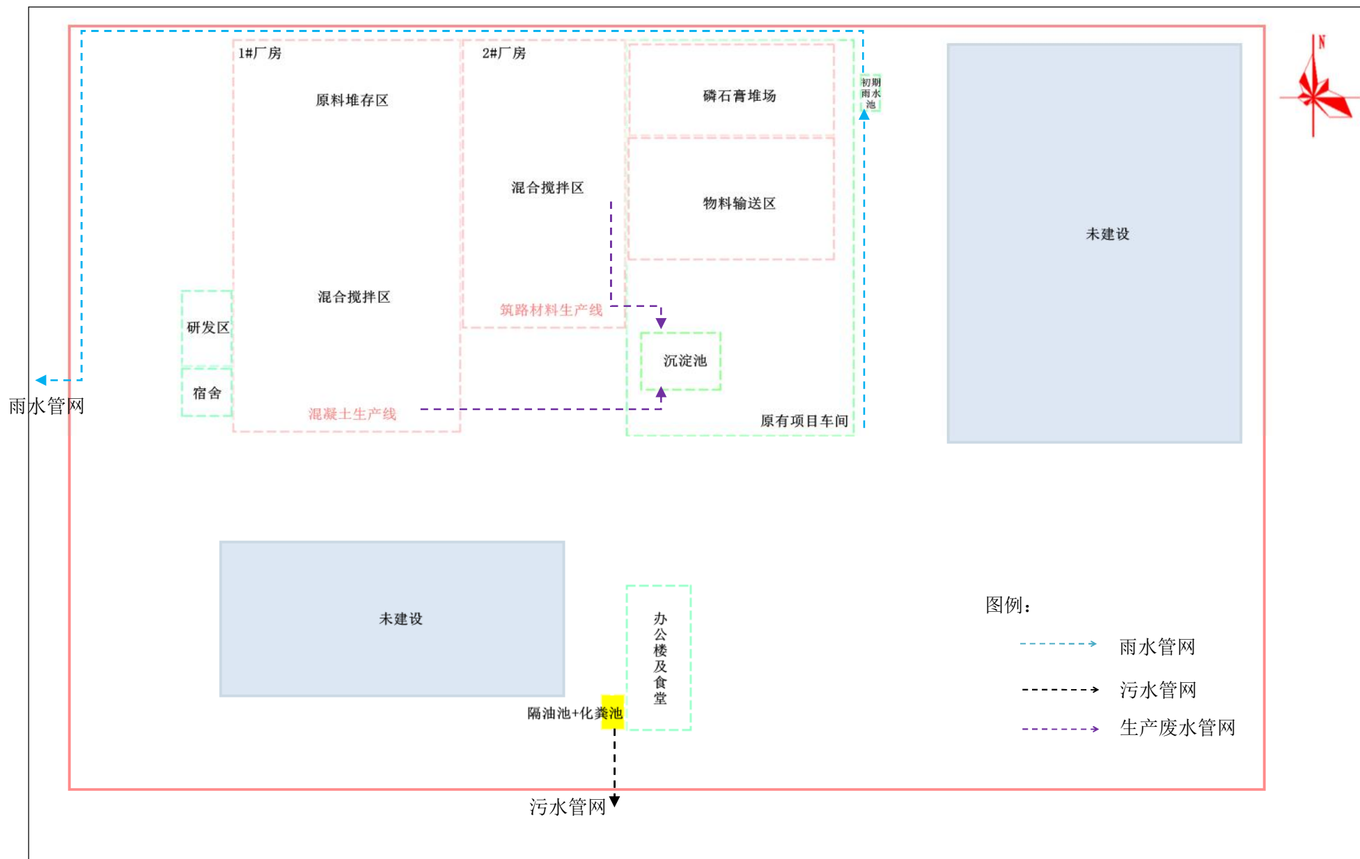
附图3 项目平面布置及雨污管网图
