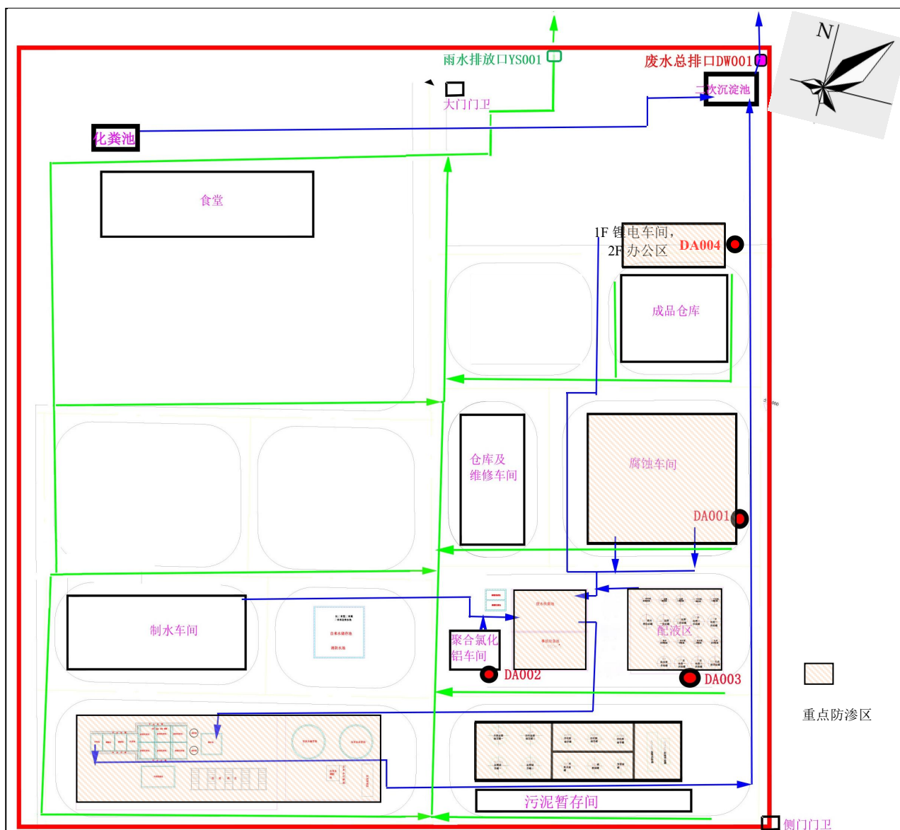
附图 4 项目厂区分区防渗图
