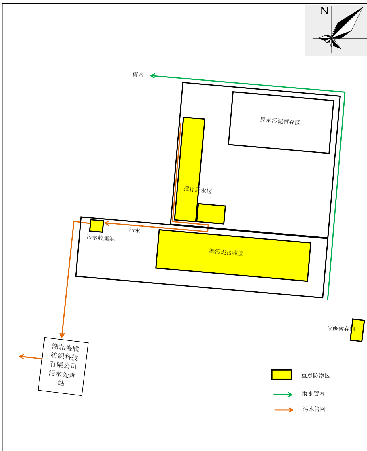
附图3 项目平面布置图及雨污管网图
