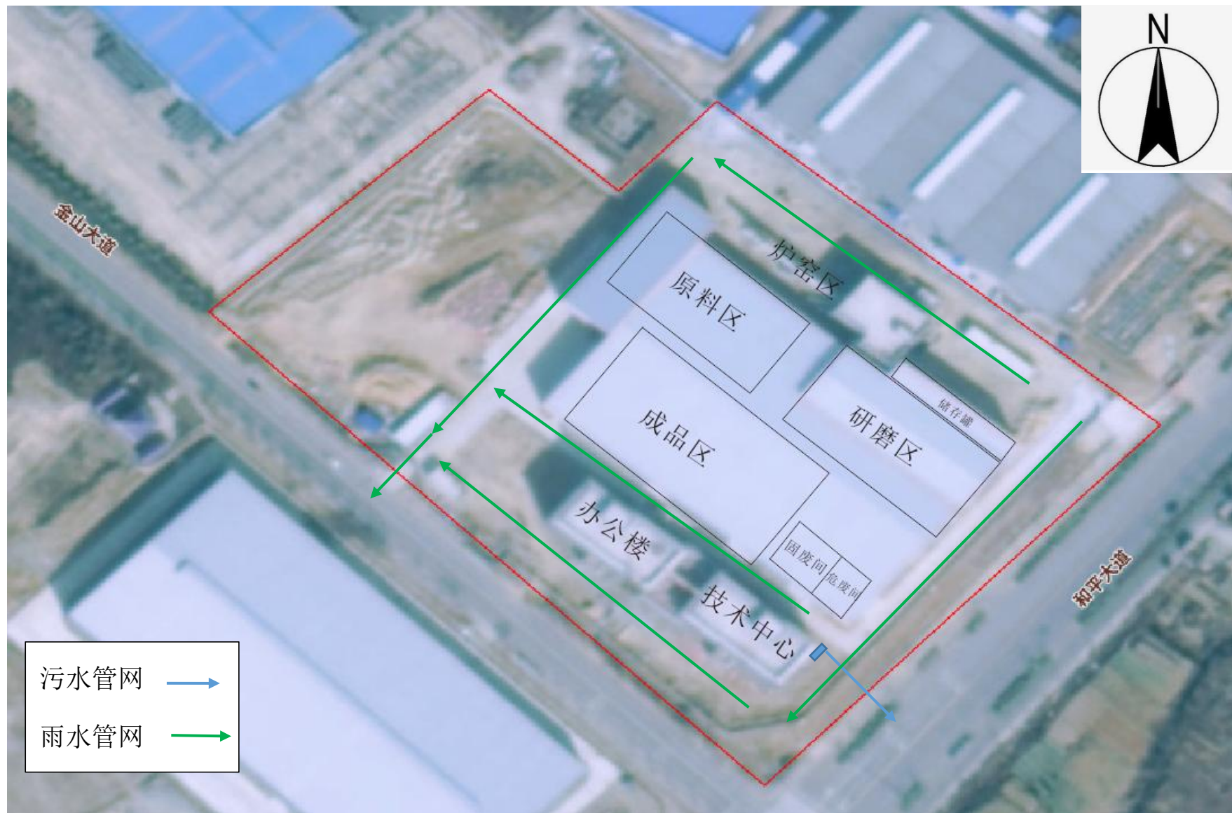
附图3 项目平面布置及雨污管网图
