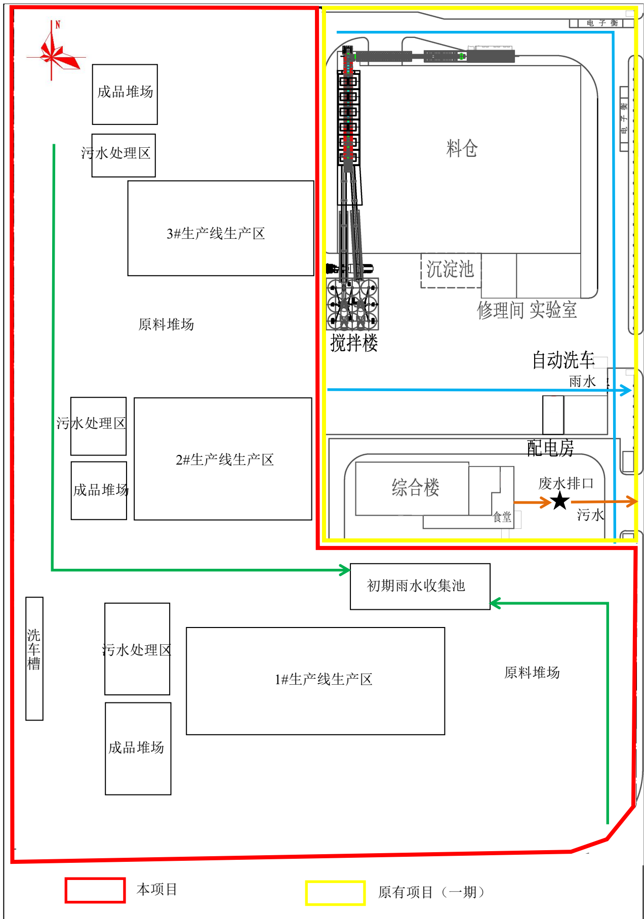
附图3 项目厂区平面布置图及雨污管网图
