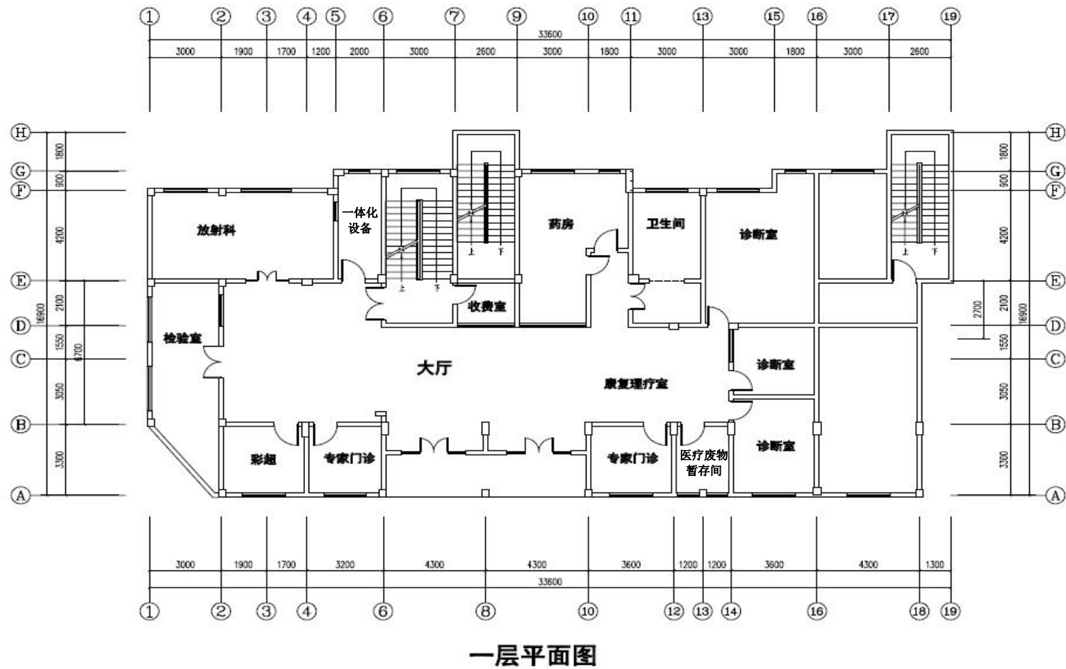
附图 3-1 项目一层平面布置图
