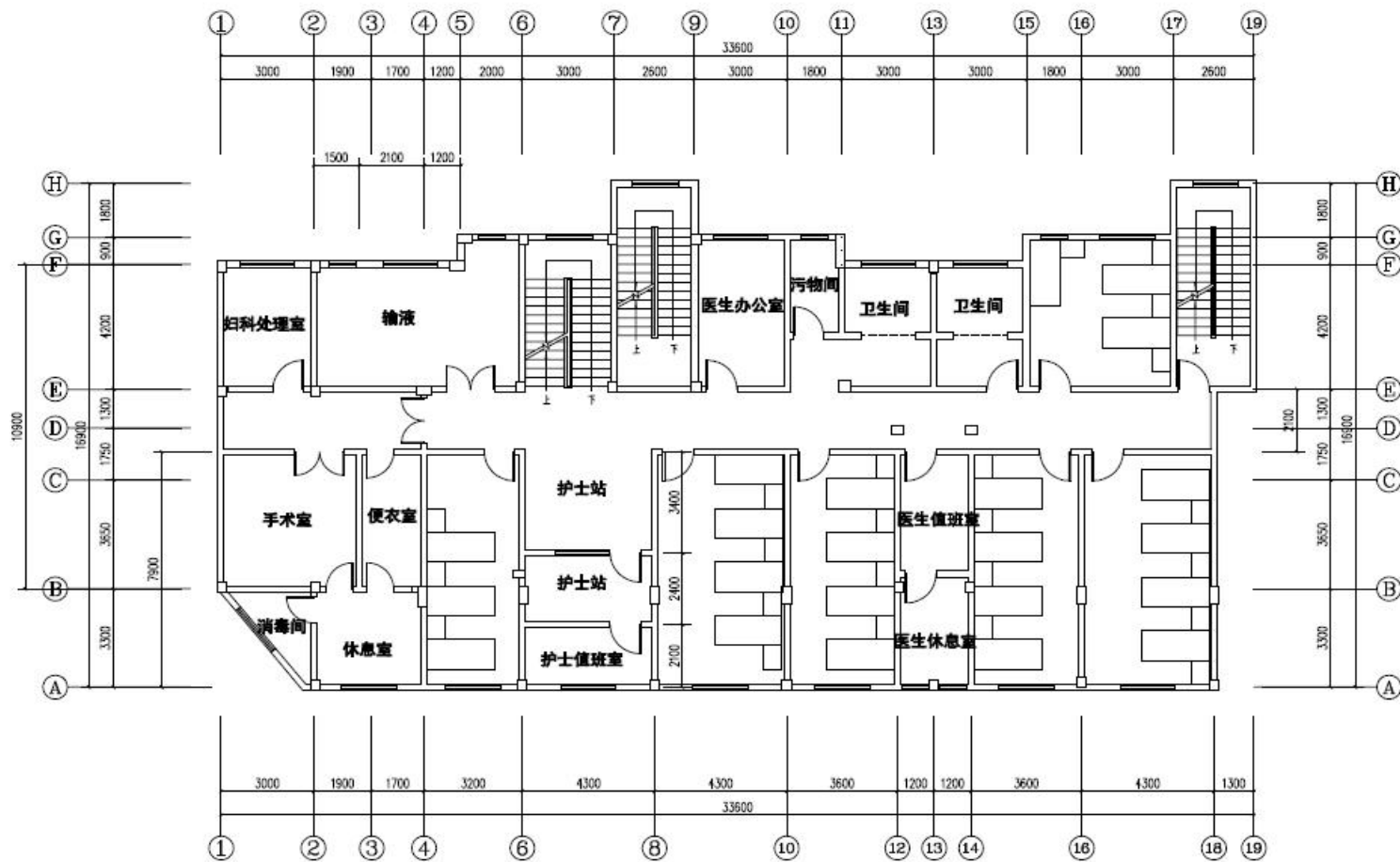
二层平面图
