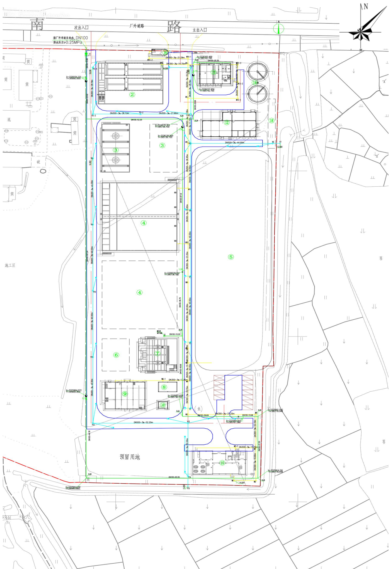
附图 6 项目雨水管网图
